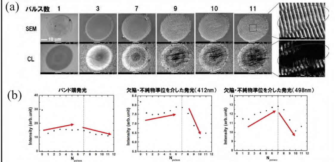
FIG. (a) GaN基板表面にレーザーパルス照射した箇所の電子顕微鏡像（上段）と電子線励起発光（CL）像（下段）。加工痕にはナノ周期溝構造が形成されていく様子が見られるが、照射パルス数を増やすにつれて全体的にCL強度が低下することから結晶構造が崩れて行っていると考えられる。(b)レーザーパルス照射した箇所のCLスペクトルから得られたバンド端発光および欠陥・不純物準位を介した発光強度のパルス数依存特性。結晶構造の変化に加え、 V_{\text{Ga}}O_{\text{N}} の複合欠陥が関連する498nmのCL変化より、酸化が進んでいると考えられる。
