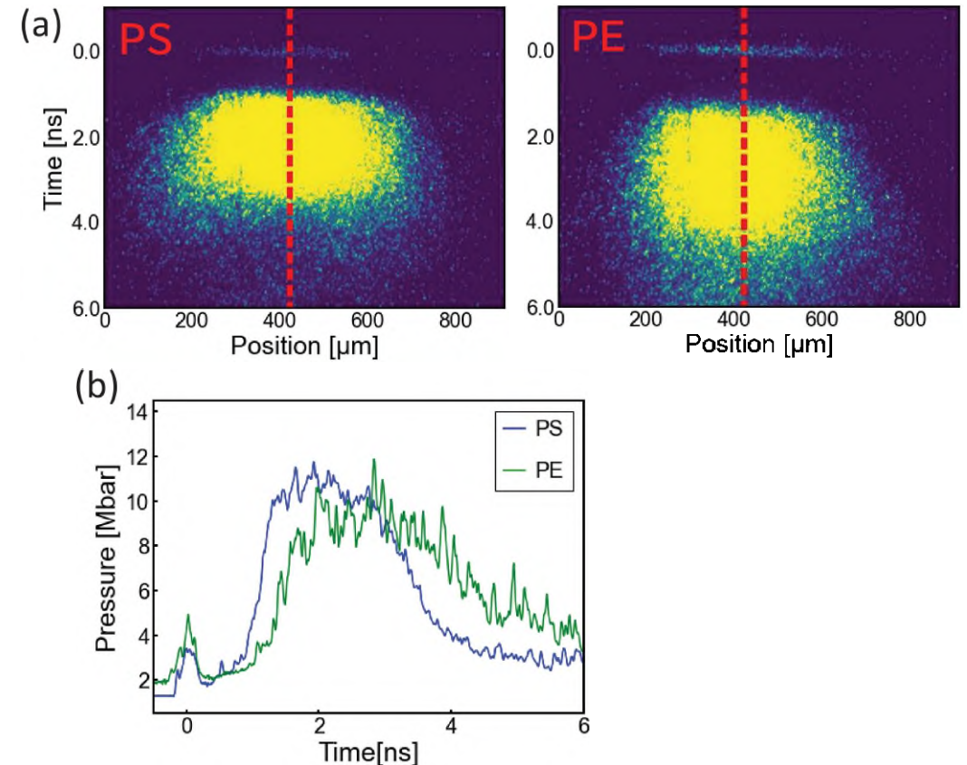
FIG. (a)輝度温度計測によるポリスチレン(PS)およびポリエチレン(PE)の衝撃波面温度計測結果. (b)それぞれの衝撃波面圧力の時間変化
