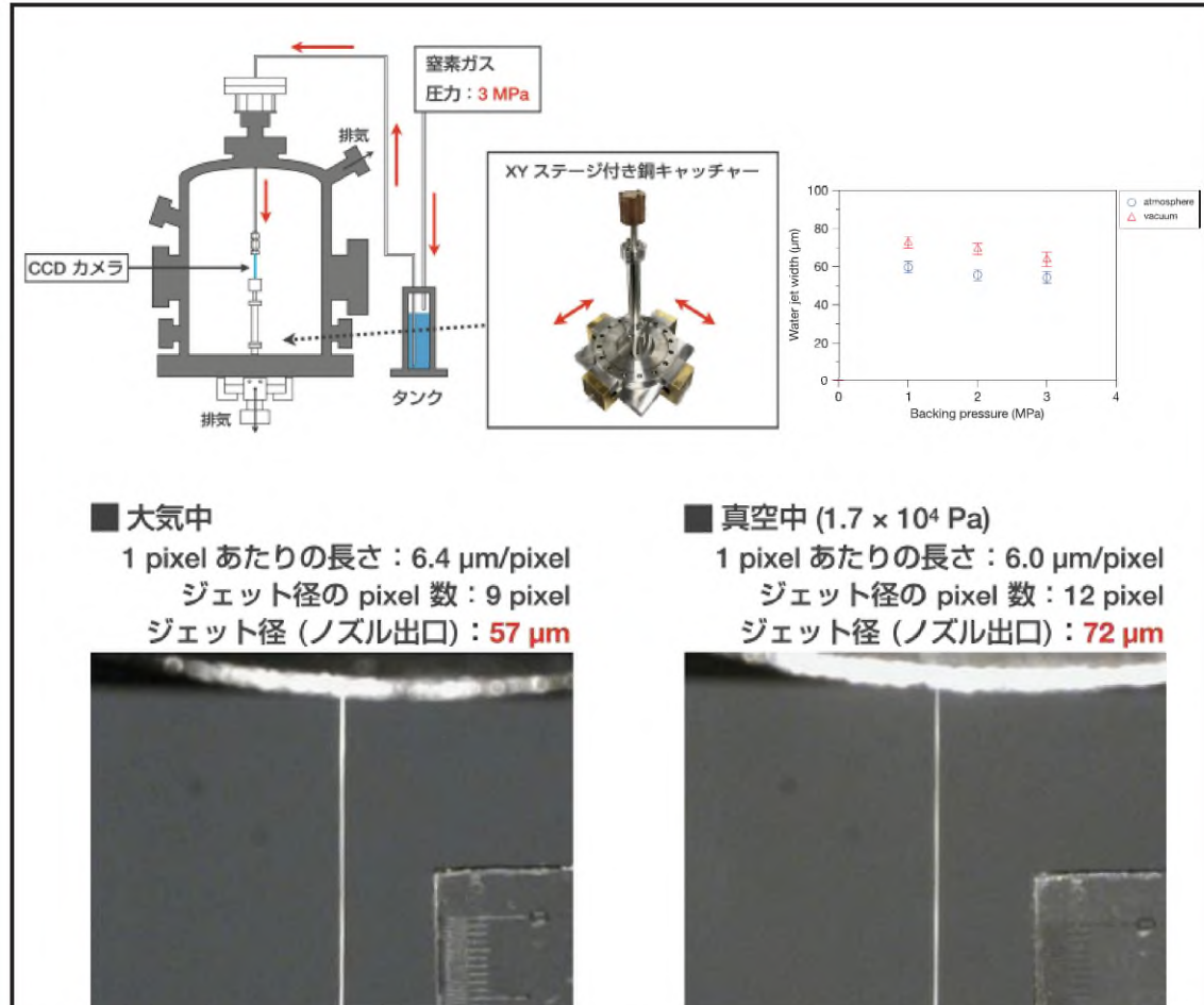
FIG. 大気中と真空中での水ジェット噴出試験の写真とジェット径の背圧依存性
