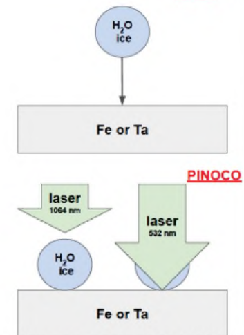
FIG. (左上) 超高速微粒子の衝突生成物、(右上) 氷微粒子のタンタル標的衝突の模擬計算、(左下) 衝突生成物に関するレーザー照射強度と微粒子衝突速度の相関性の概念図、(右下) iSALEとPINOCOコードの計算モデル。
