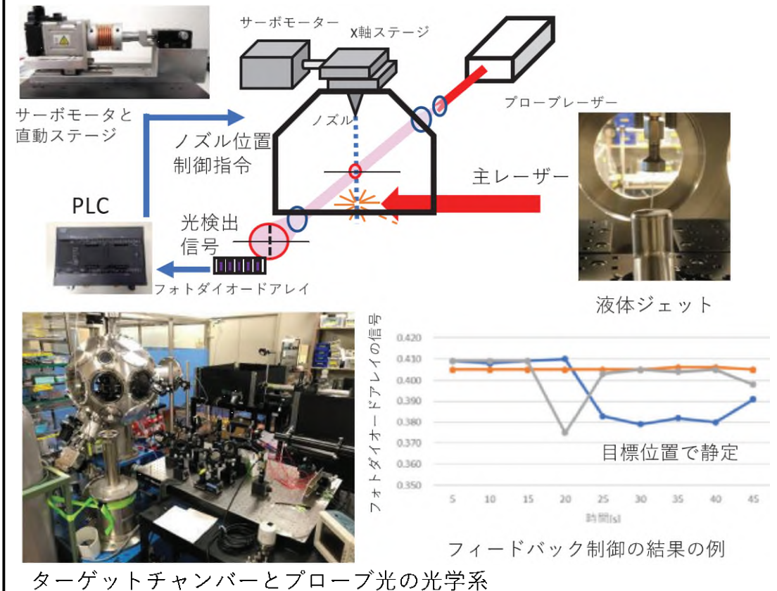
図1 液体ジェットによるターゲット位置のフィードバック制御実験系の概要と、フィードバック制御により目標位置で静定させることができることを確認した。
