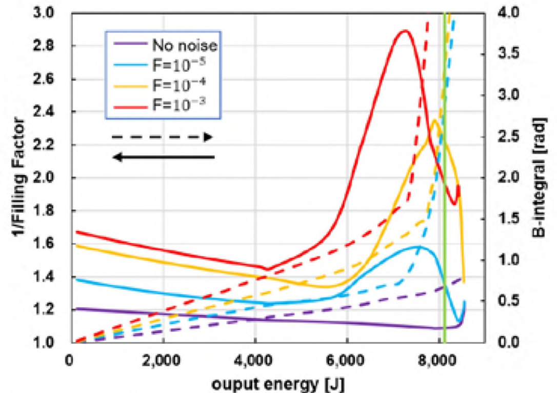
FIG. output energy と 1/Filling Factor と B-integral
