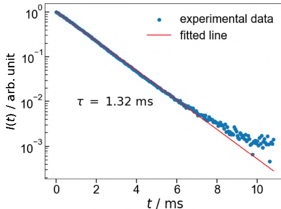
FIG. Ba 3 Y 2 O 5 Cl 2 :Eu4 %の 5 D 0 → 7 F 2 遷移の蛍光寿命(励起 250 nm)
