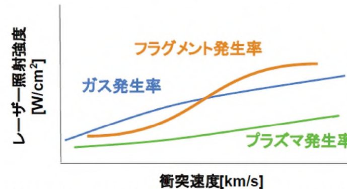
FIG. (左上) 超高速微粒子の衝突生成物、(右上) 氷微粒子のタンタル標的衝突の模擬計算、(左下) 衝突生成物に関するレーザー照射強度と微粒子衝突速度の相関性の概念図、(右下) iSALEとPINOCOコードの計算モデル。
