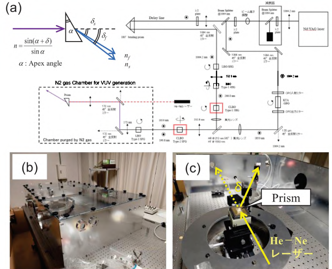
FIG. (a) 測定系の概要。
