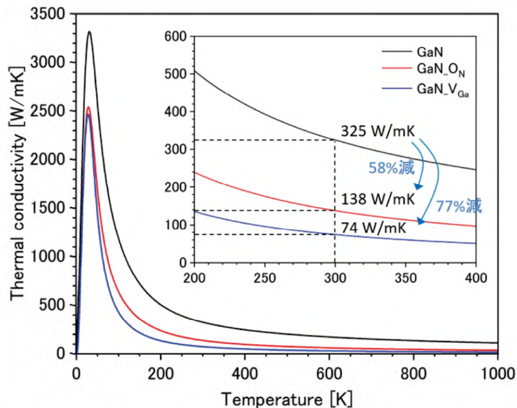
FIG. 1 GaNの熱伝導率の温度依存性。O N はN原子をO原子に置換したO欠陥モデル、またV Ga はGa空孔モデルである。欠陥濃度は約 1.3 \times 10^{21} cm -3 に相当する。同位体散乱と寸法効果（1mm）を考慮している。
