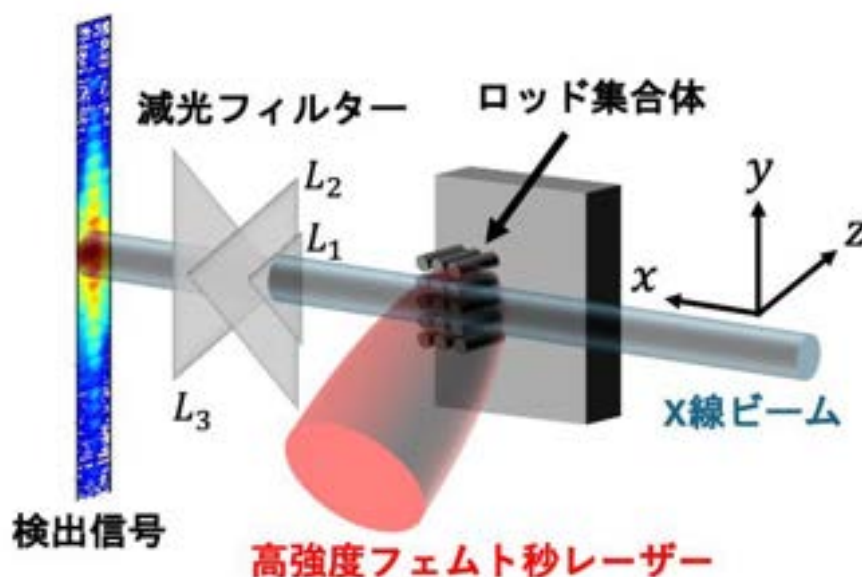
図1. 高強度フェムト秒レーザーによる微細ロッド集合体ターゲットのプラズマ化ダイナミクスに対するX線自由電子レーザーを用いた観測実験の概念図。
