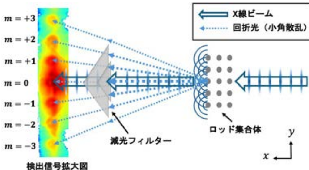
図2. ビームストップフリーX線小角散乱法の原理図。検出信号の左に記載されている m は回折次数を表す。本実験で用いた減光フィルターは、一定の厚みをもつ三角形形状の金属薄板を重ね合わせることで、中心部ほど厚くなるように構成される。フィルターを三角形形状にすることで、重ね合わせる位置に応じて減光領域を細かく調整することが可能。
