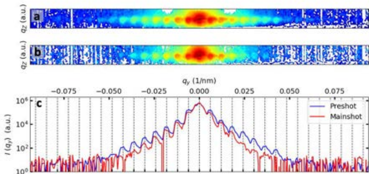
図3. 実験結果。減光フィルターの既知の透過率を用いて、各領域の信号強度を補正した画像（検出信号）。(a) 固体状態の円柱集合体ターゲットからの小角散乱信号。横軸の q_y は y 方向の回折角度に対応する波数。(b) 励起光照射から 7.5 ピコ秒後のプラズマ化した円柱集合体ターゲットからの小角散乱信号。(c) a と b の一次元投影強度分布を重ねたプロット。
