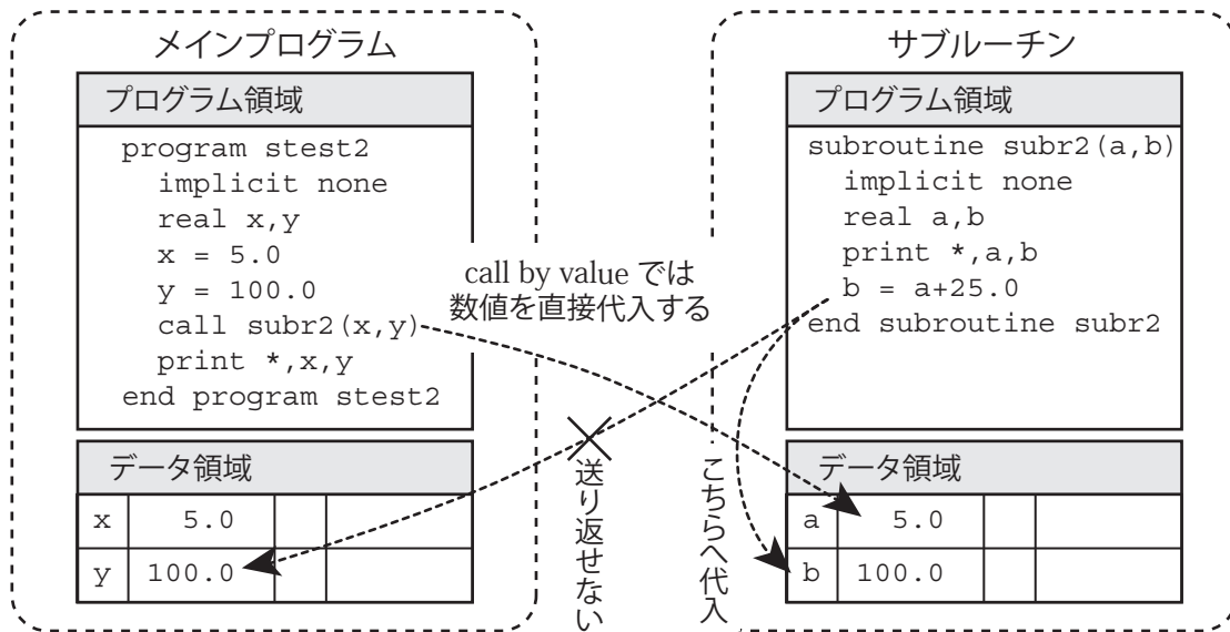
図 3.3 “call by value”を使ったデータ渡しでは値を送り返さない
