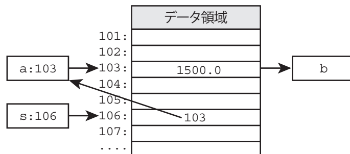
図 3.5 間接アドレスによるメモリ参照
