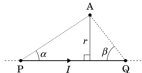
図 1.4 線分電流
